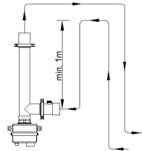
vertikaler Einbau
