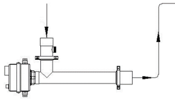
horizontaler Einbau
