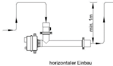
horizontaler Einbau
