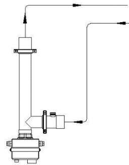
vertikaler Einbau
